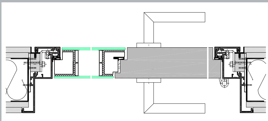
Glasverbund-Seitenteil Typ GVF-S in Aluminiumzarge Typ USBA-G hardline
